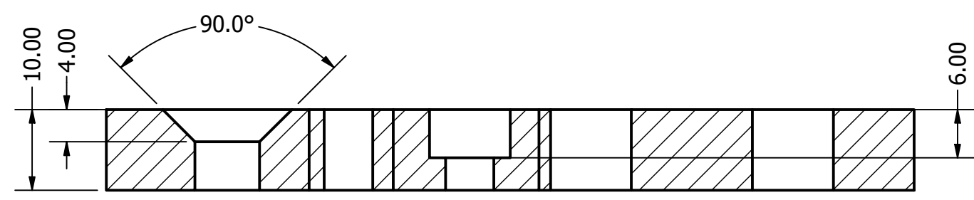
SECTION A-A SCALE 1.5 : 1
