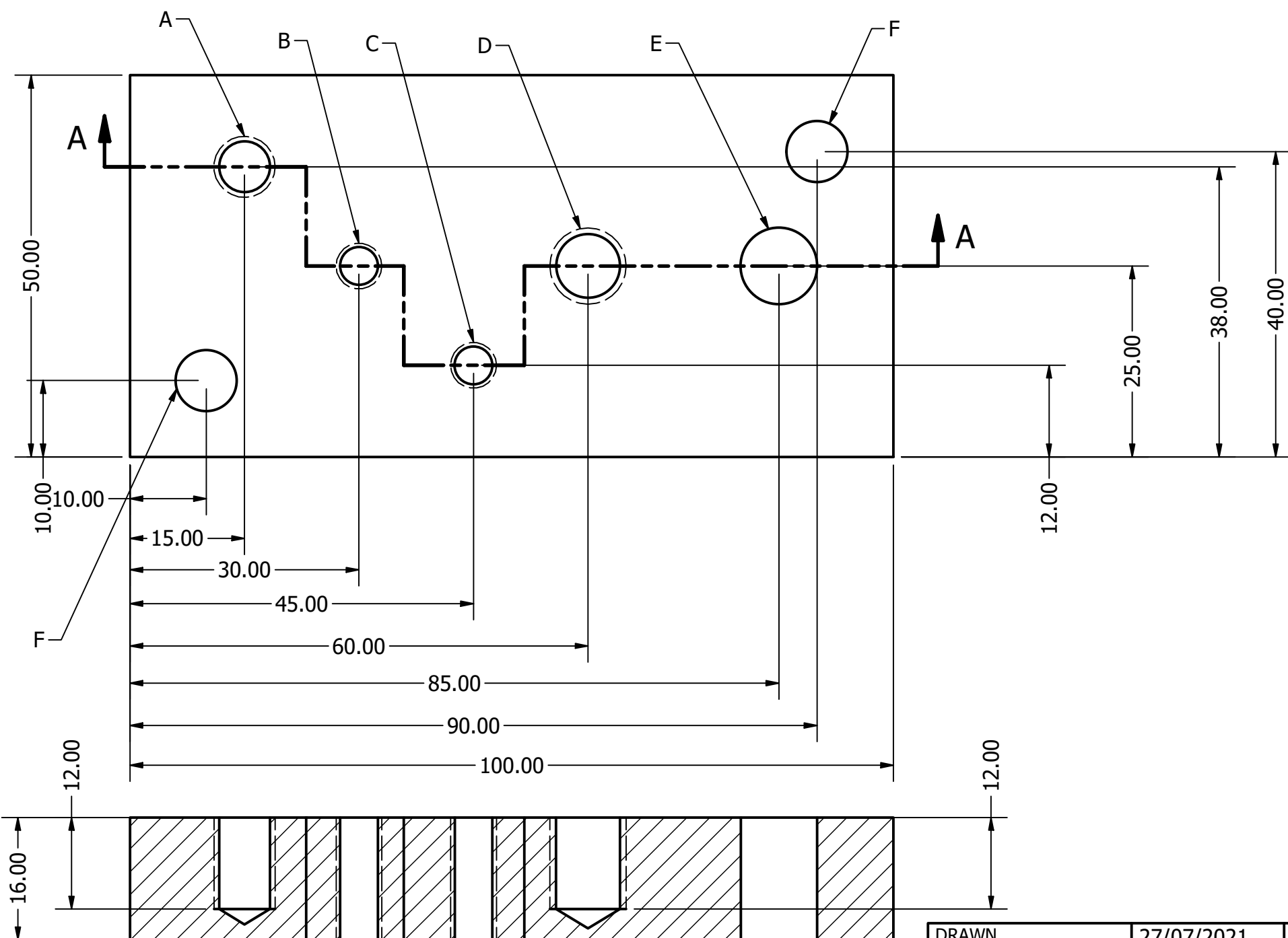
SECTION A-A SCALE 1.5 : 1
